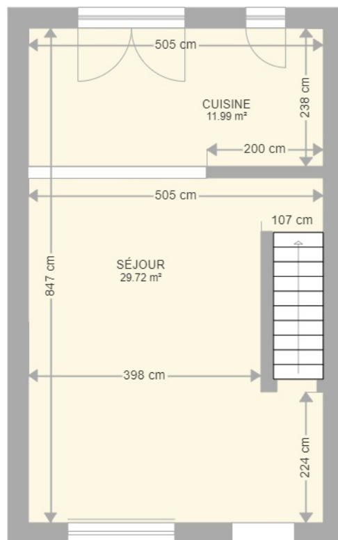
Rez-de-jardin
