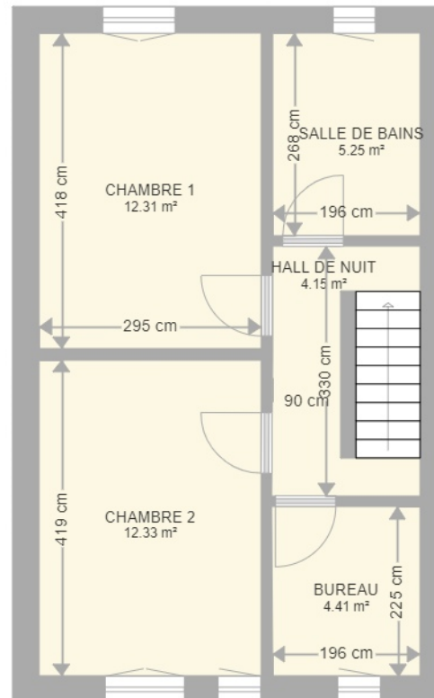
1er étage
